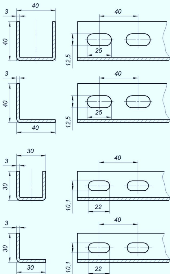
Профиль U, L - обр. оцинкованный толщина 3 мм
