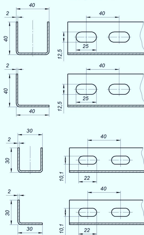
Профиль U, L - обр. оцинкованный толщина 2 мм
